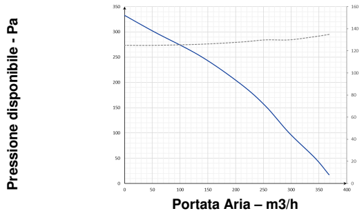
PRESTAZIONI AERAUICHE INTEGRAZIONE/DEUMIDIFICA
