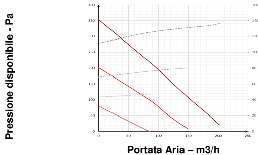
PRESTAZIONI AERAUICHE VENTILAZIONE
