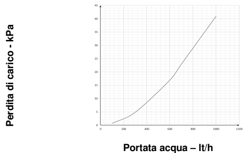
PERDITA DI CARICO/PORTATE BATTERIA IDRONICA
