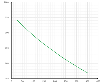
EFFICIENZA TERMICA ESTIVA (2)
